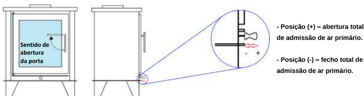
Figura 2. Exemplo de abertura da porta e manipulação do registo de ar primário
