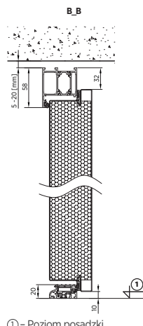
Przekrój pionowy drzwi THOR.
