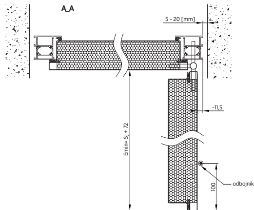
Przekrój poziomy drzwi THOR.
