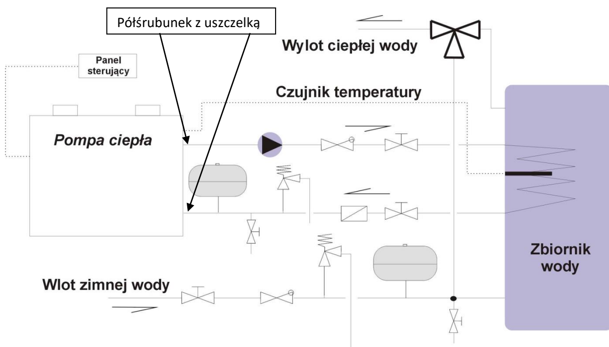
Rys. B Schemat podłączenia pompy ciepła do zbiornika wody – podłączenie do węzownicy zbiornika cwu.
