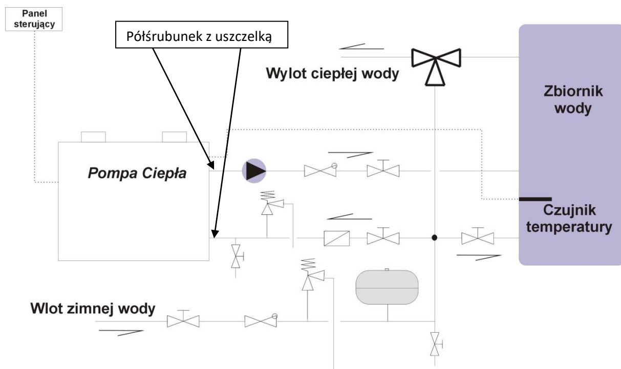
Rys. A Schemat podłączenia pompy ciepła do zbiornika wody – podłączenie w obieg wody wodociągowej – cyrkulacyjnej.
