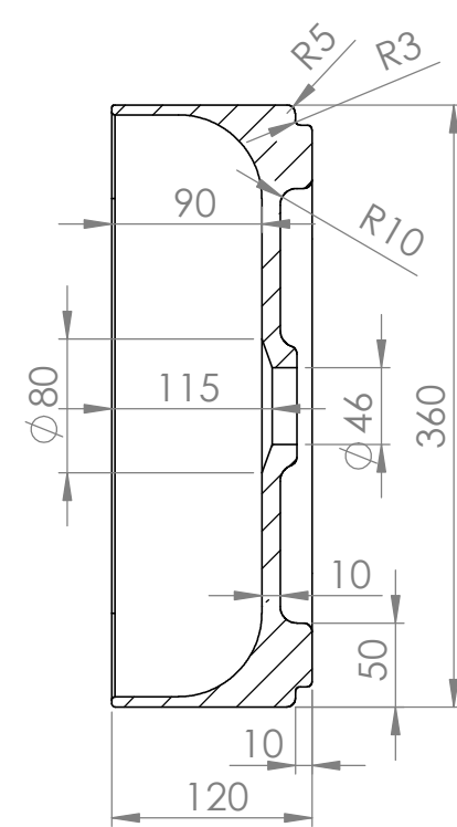
SECCIÓN C-C
