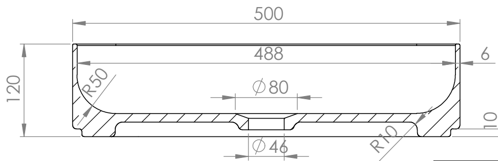
SECCIÓN B-B
