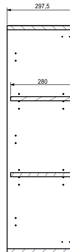
A-A ( 1 : 10 )
