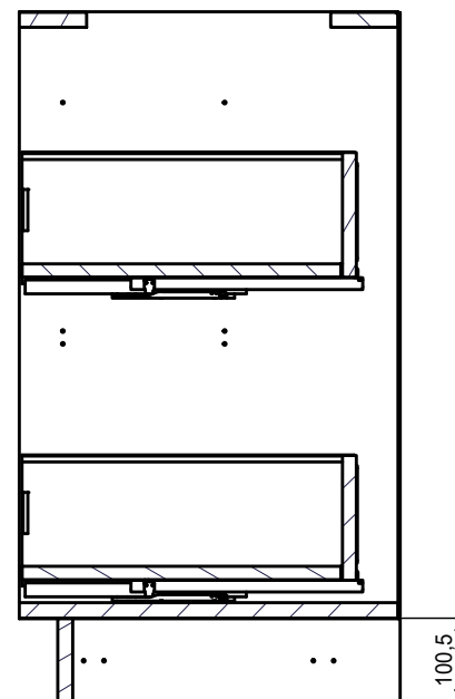
A-A ( 1 : 10 )
