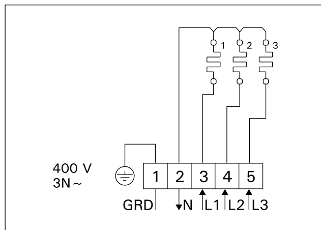
Figura 11. Conexiones eléctricas (BC-E)
