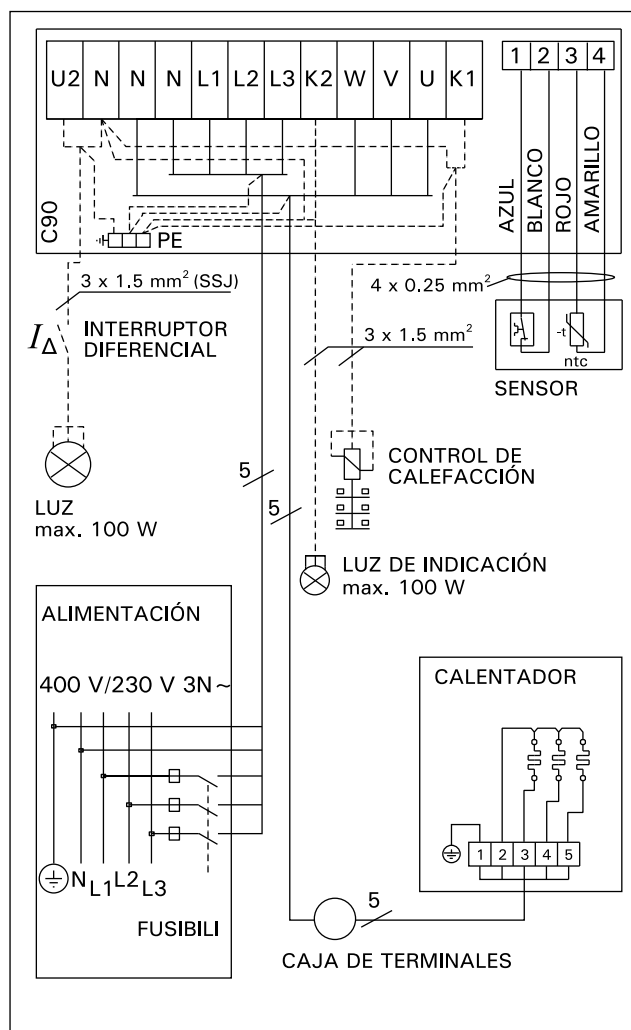
Figura 12b. 3-fase conexión (centro de control C90 + BC-E)
