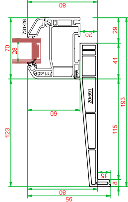
Coupe pièce d'appui de base
