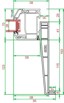
Coupe pièce d'appui de base
