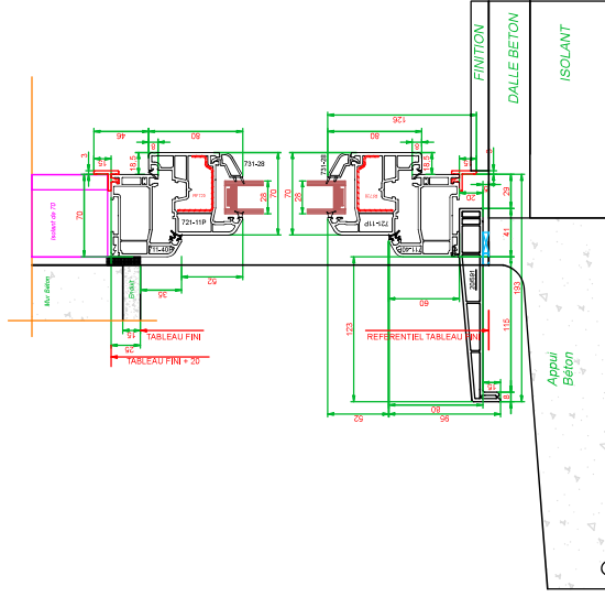
Coupe définition de base B-B
