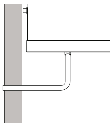
fig. 57 - Ejemplo de conexión del drenaje de condensado sin sifón
