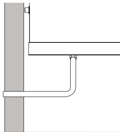
fig. 57 - Exemplo de ligação da drenagem da condensação sem sifão
