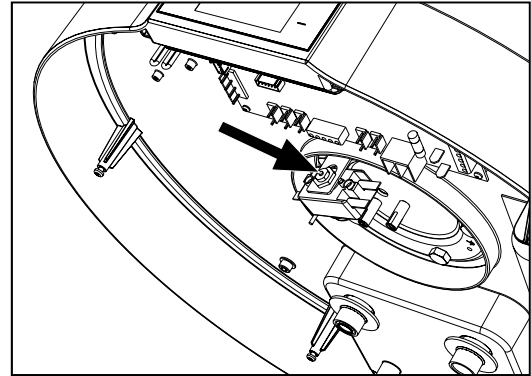
fig. 65 - Rearme del termostato de seguridad
