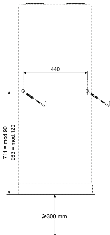
fig. 50 - Indication de perçage
