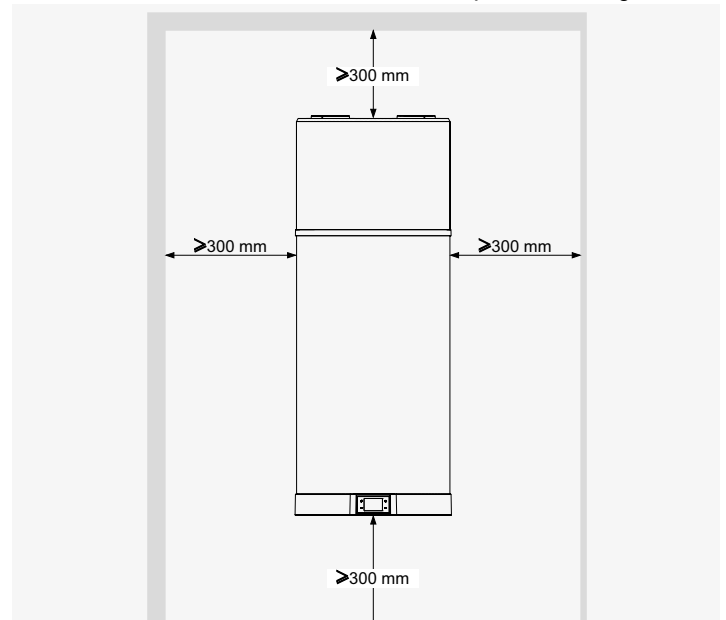
fig. 49 - Espaces minimum
