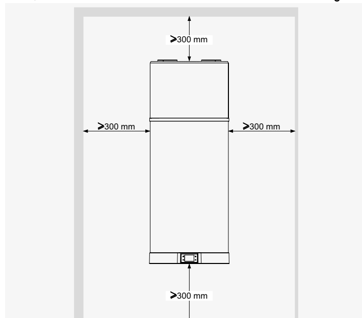
fig. 49 - Espaços mínimos
