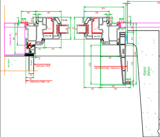
Coupe définition de base B-B
