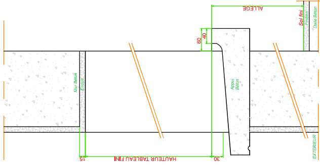
Coups pièce d'appui de base
