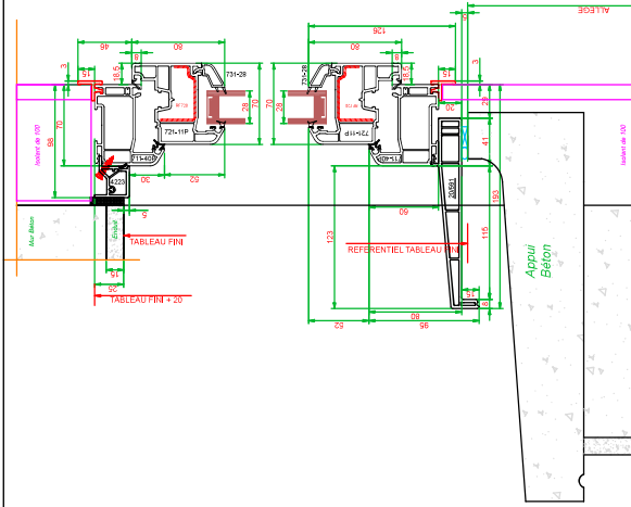
Coupe définition de base B-B
