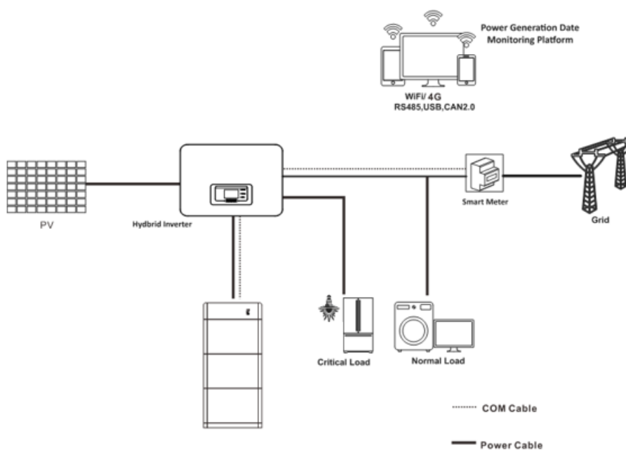
Figura 3 – Schema del principio di applicazione AZZURRO ZT-ZBT5K-ES5 ~ ES20
