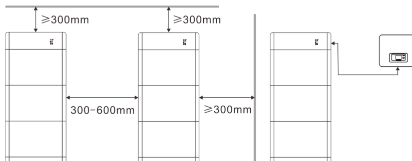
Figura 9 - Spazio di installazione
