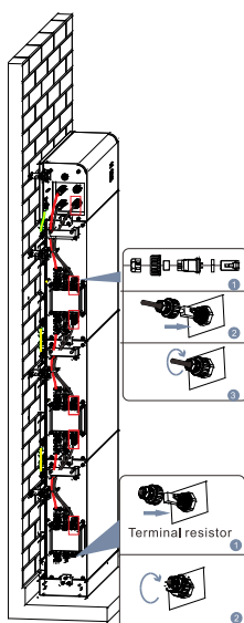
Figura 17 - Collegamento dei cavi di segnale interni
