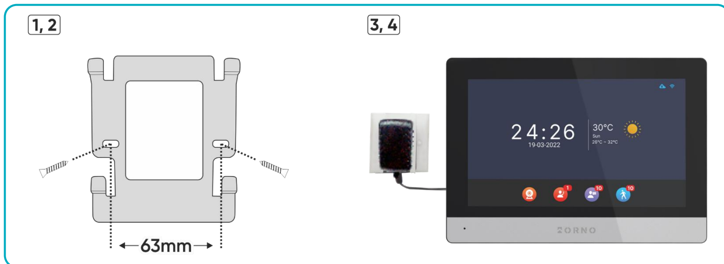
rys. 3 Montaż monitora
