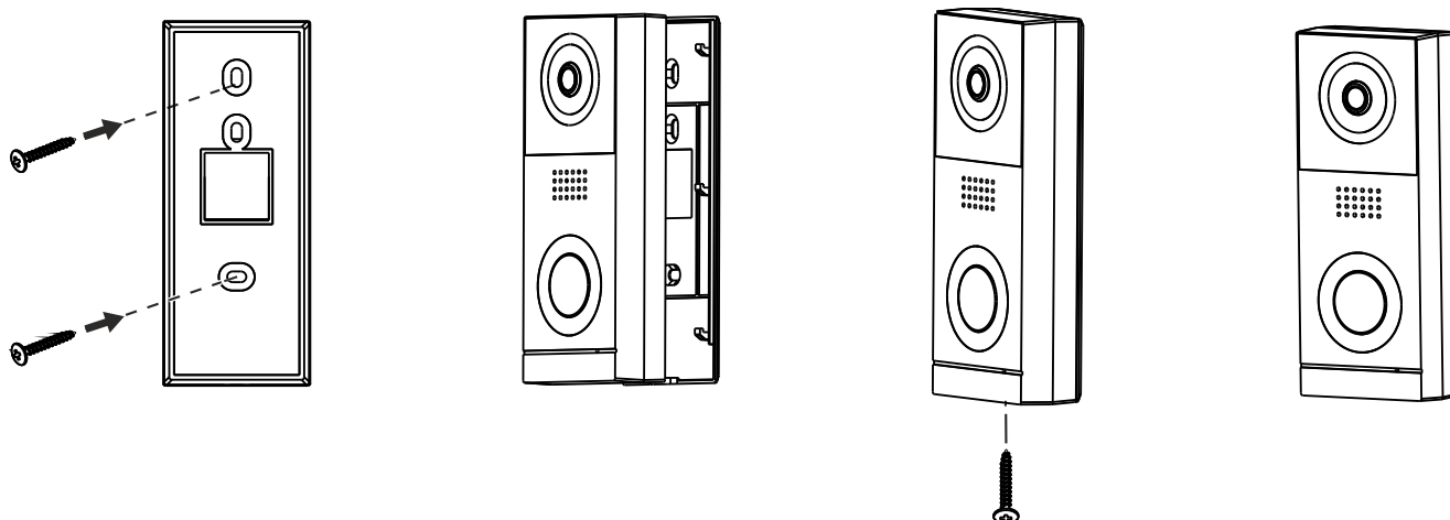
rys. 5 Montaż panelu zewnętrznego
