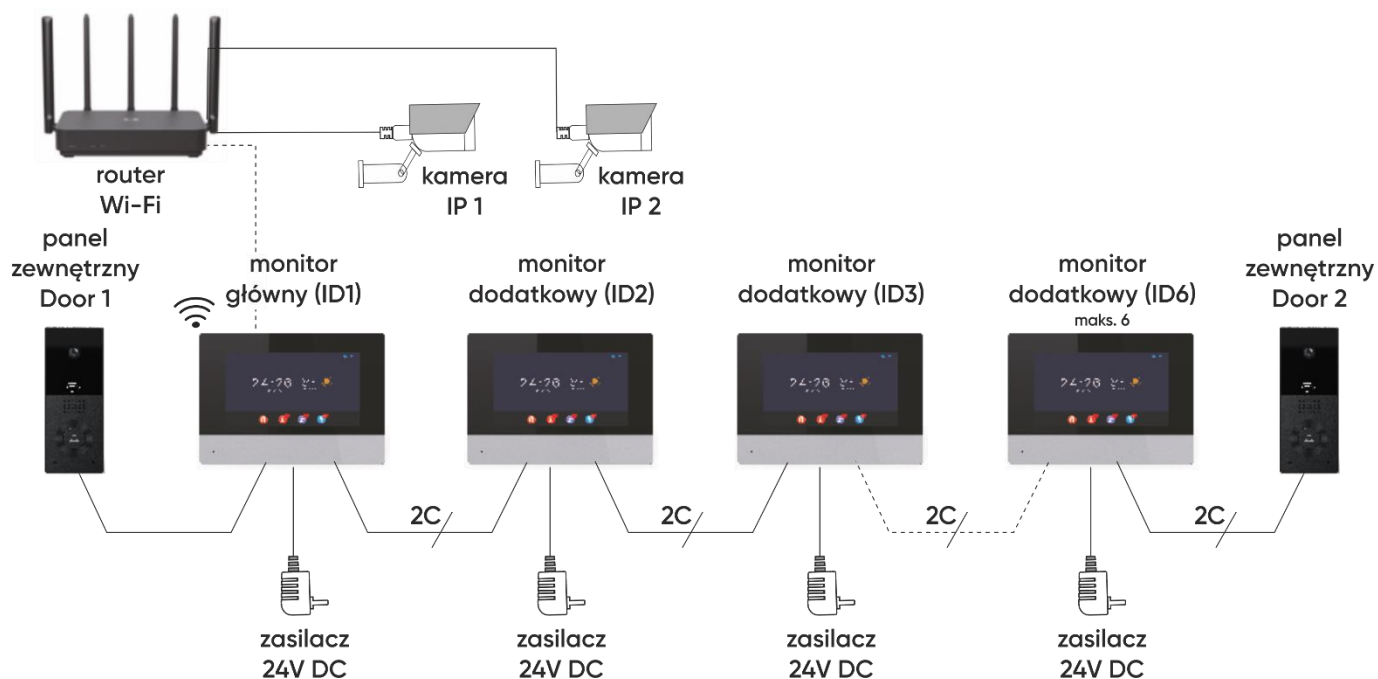
rys. 6 Schemat podłączenia
