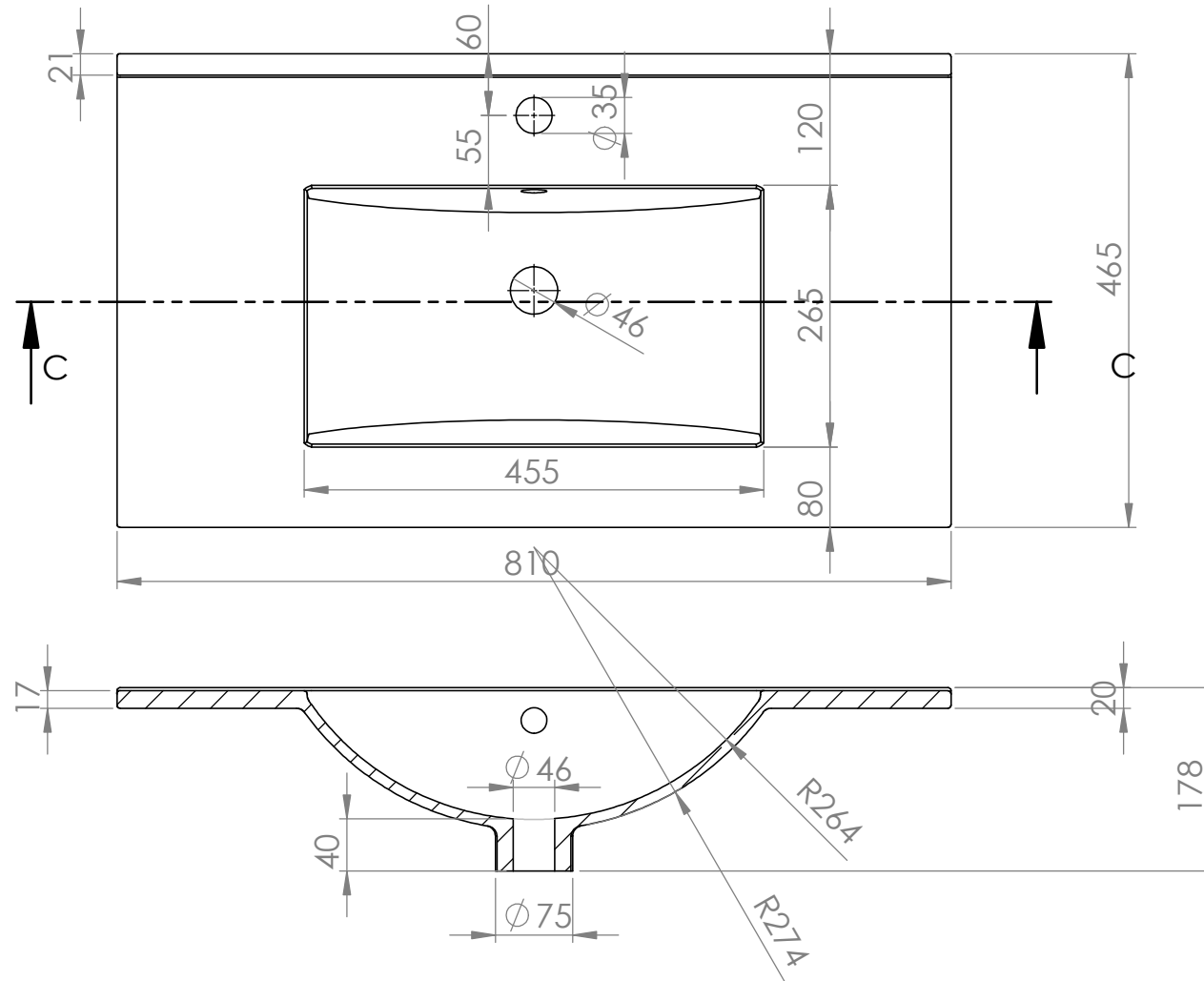
SECCIÓN C-C
