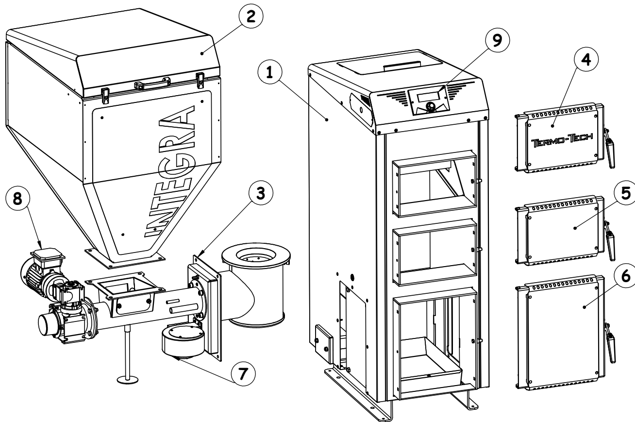
1-korpus, 2- zbiornik paliwa, 3- podajnik paliwa, 4-drzwiczki wyczystne, 5-drzwiczki wyczystne, 6- drzwiczki popielnikowe, 7-wentylator, 8-motoreduktor, 9-sterownik
