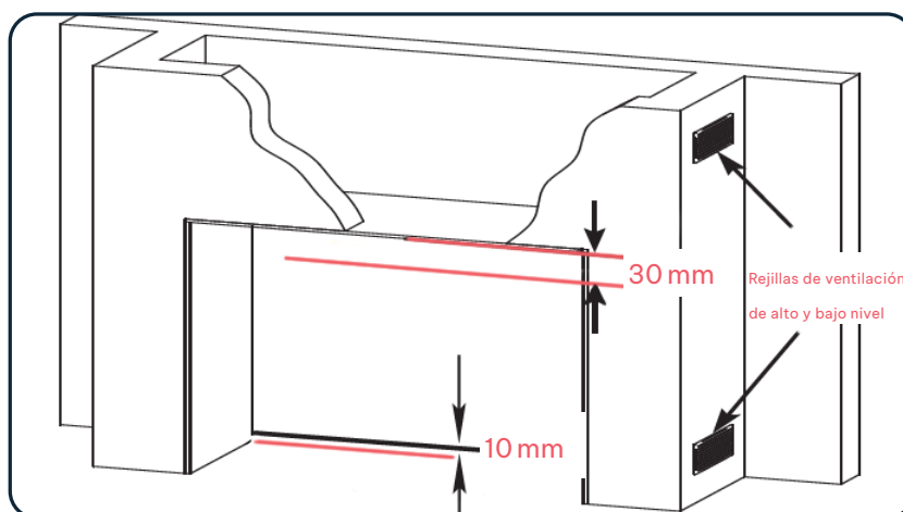
INSTALACIÓN DE CONDUCTO DE HUMOS ABIERTO
