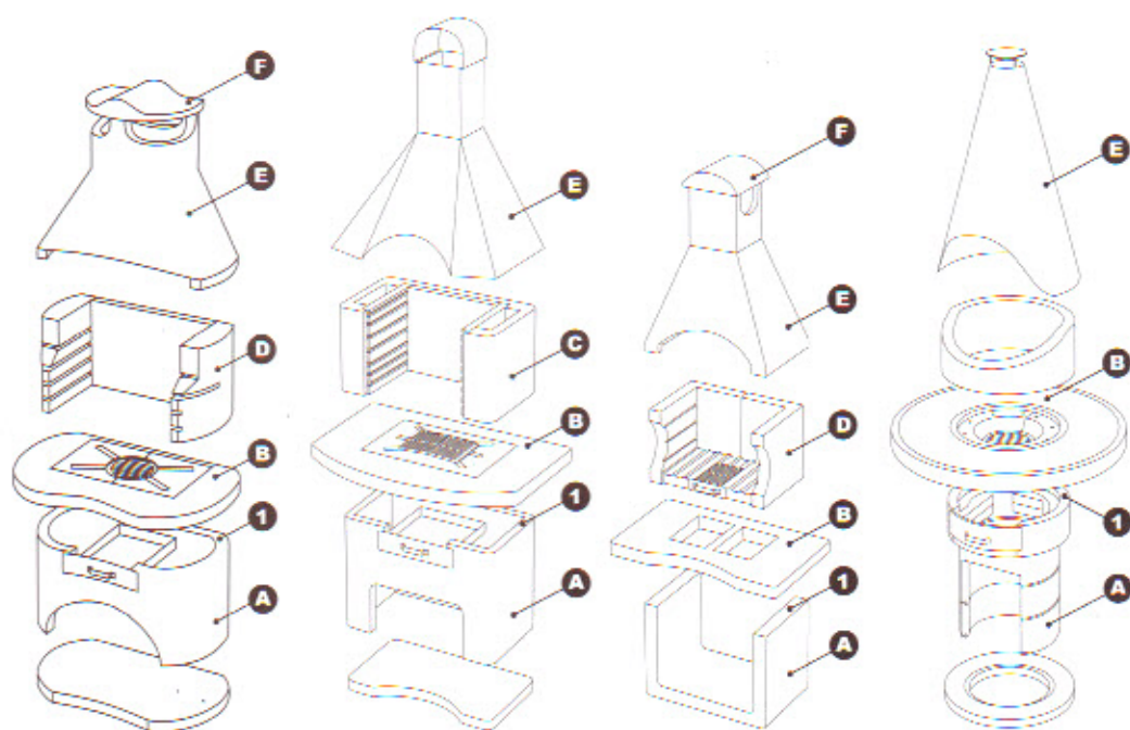
A - podstawa, B - płyta stołowa, C,D - palenisko, E - okap, F - daszek
