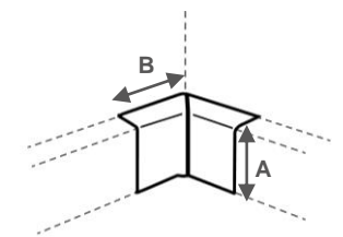
Angle intérieur
