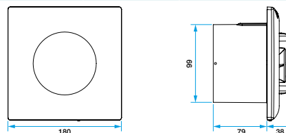
Encadrement en mm
