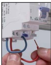
Réaliser le câblage
