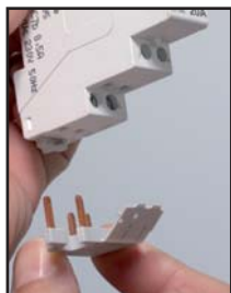
Dévisser le connecteur
