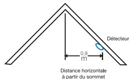
Schéma 5 : Montage en sous-pentes
