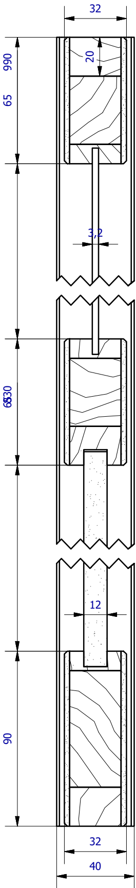
C-C ( 1:2 )
