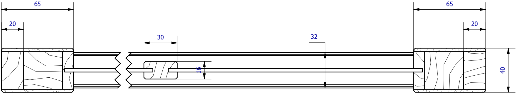
A-A ( 1:2 )
