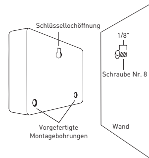
Abbildung 2: Aufhängen des Timers an der Schraube (mit der Schlüssellochöffnung)
