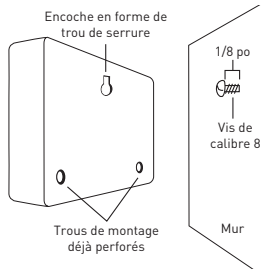
Figure 2 : Accrochez la minuterie au mur en insérant la vis dans l'encoche en forme de trou de serrure.
