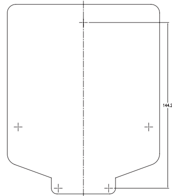
Abbildung 1: Verwenden der (mitgelieferten) Montagevorlage
