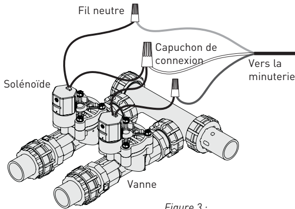
Figure 3 : Câblage des électrovannes
