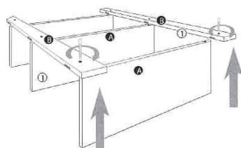
Etape 1 : Emboîter et fixer
