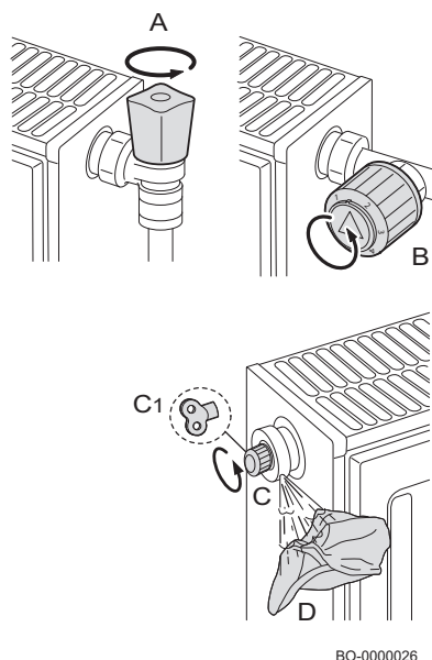
Rys.6 Przedmuchiwanie instalacji
