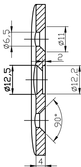
PRESJEK A-A
