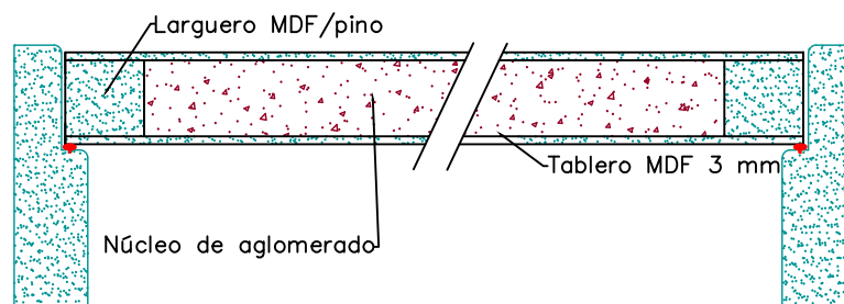
Sección horizontal (escala 1:5)
