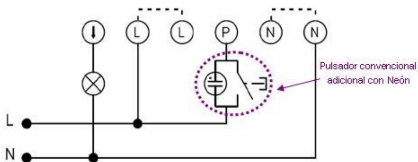
Instalación con pulsador convencional adicional:
