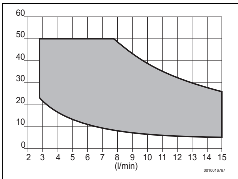
Fig. 28 Modelo 15 litros
