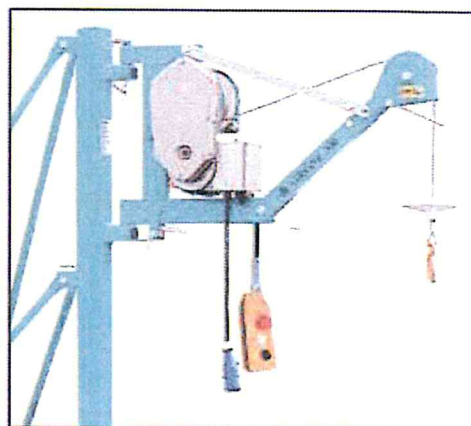
El AIRONE-300, se arriestra sobre una robusta y Certificada columna con bípode incorporado.
