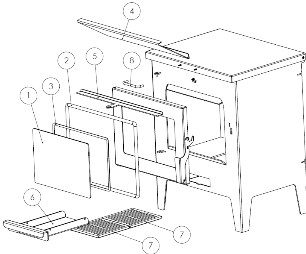
Figura nº15 - Explosionado Javea CP
