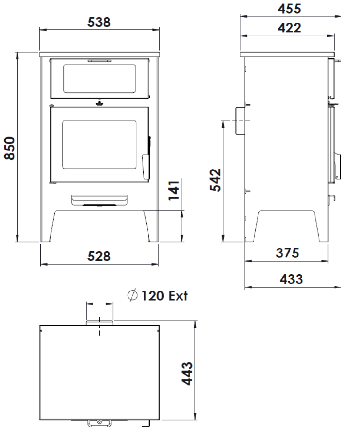
Figura n°3 - Dimensiones en mm del aparato Javea CH
