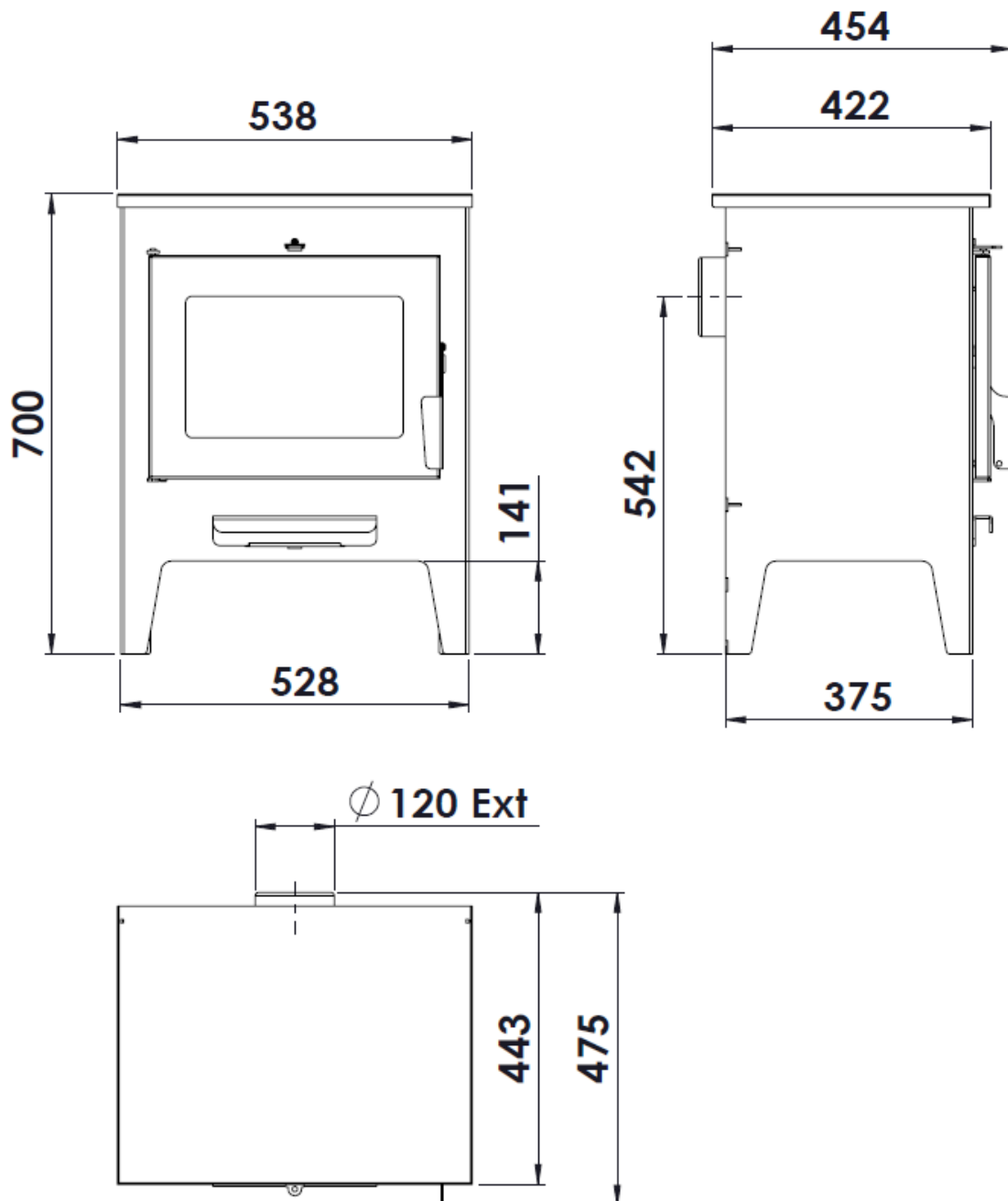
Figura n°1 - Dimensiones en mm del aparato Javea
