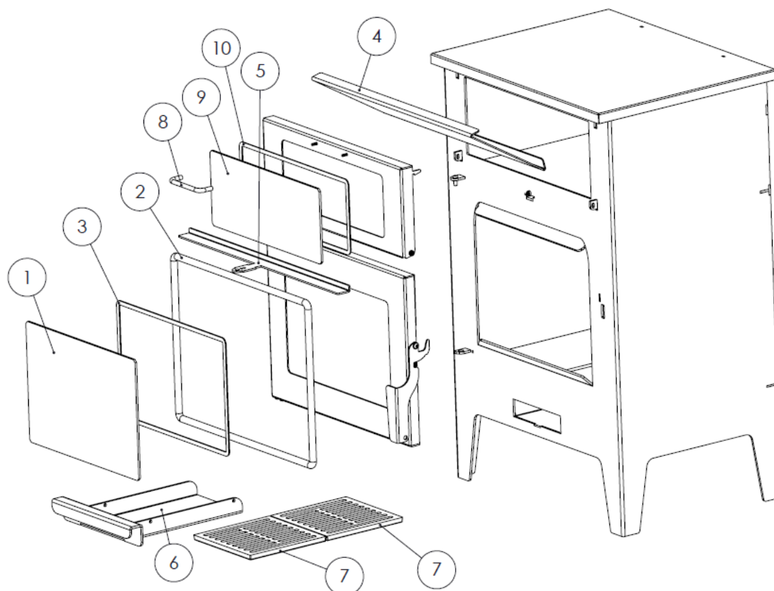
Figura nº16 - Explosionado Javea CH
