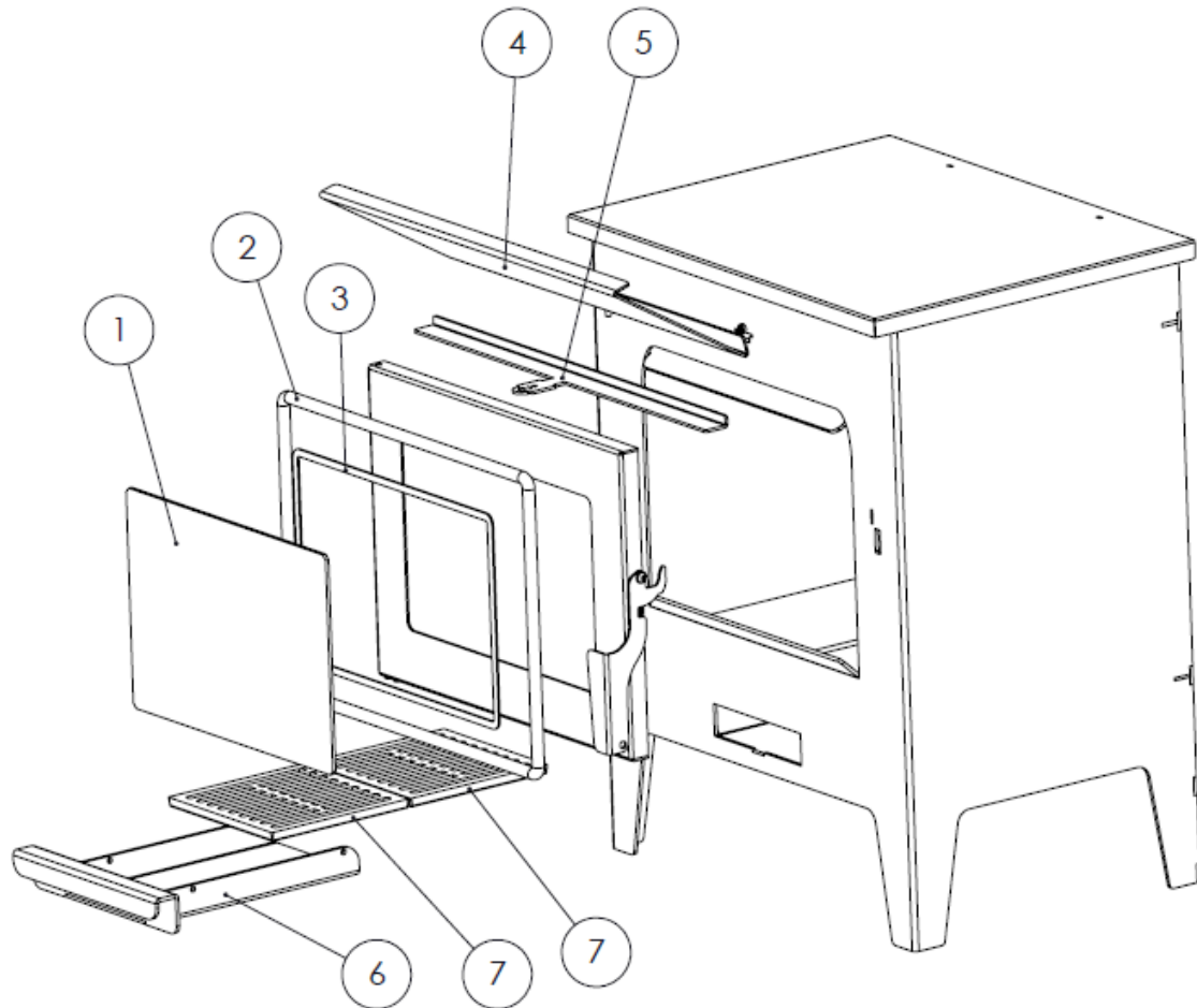
Figura n°14 - Explosionado Javea
