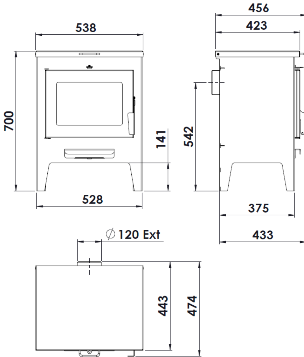
Figura nº2 - Dimensiones en mm del aparato Javea CP
