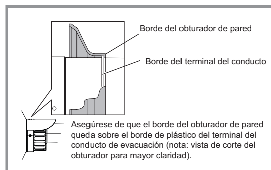
figura 16 - Obturador de pared
