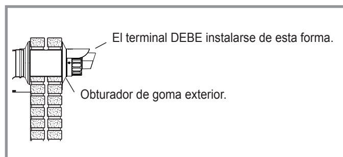
figura 17 - Conducto de evacuación y obturadores una vez instalados
