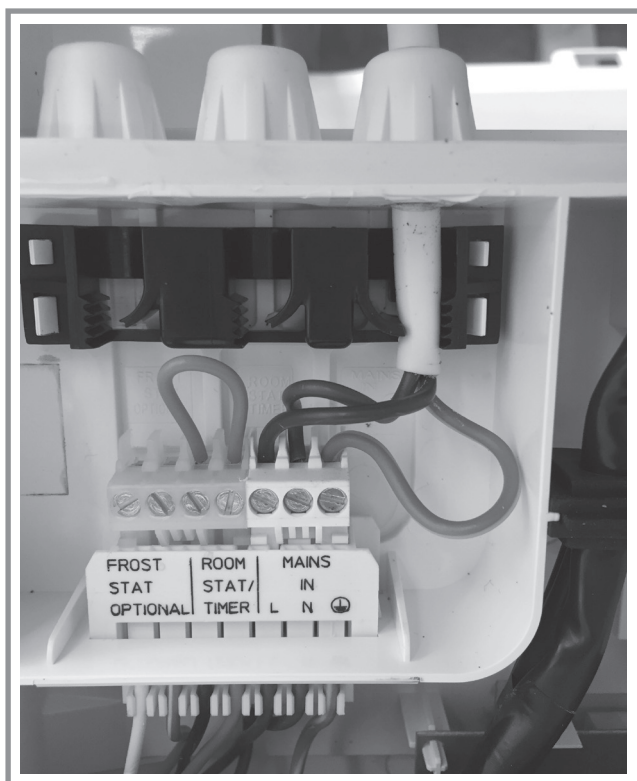
figura 33 - Conexiones preinstaladas (lado izquierdo)
