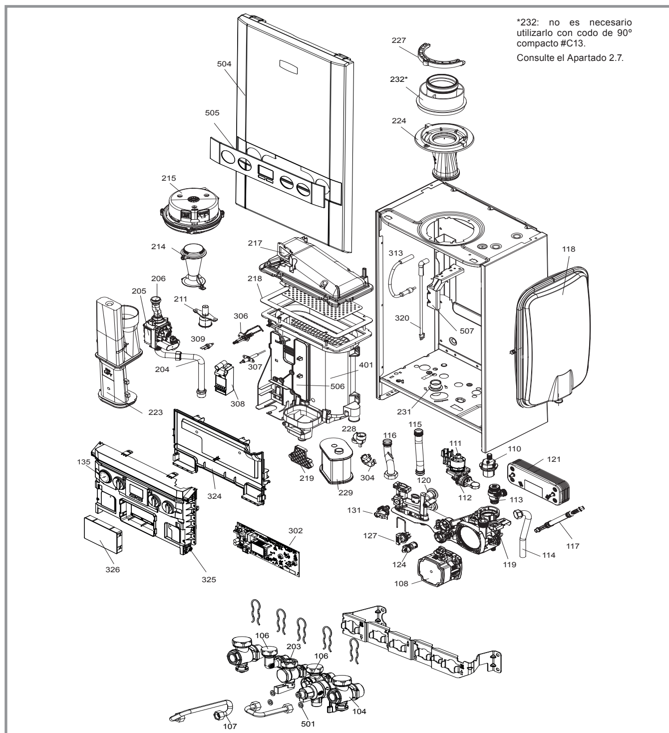
figura 4 - Ensamblaje de la caldera
