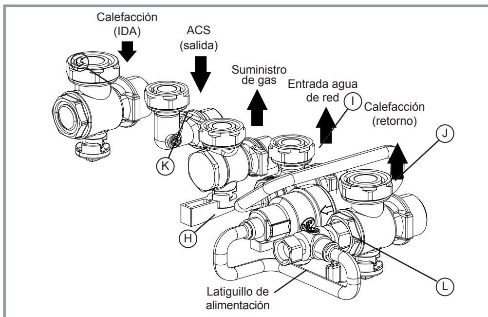
figura 38 - Conexiones de tubería
