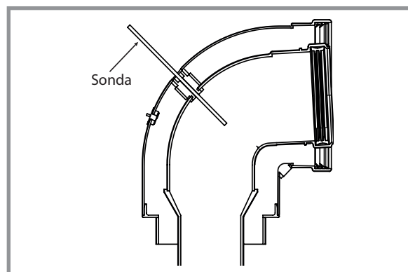
figura 22 - Medición de la presión del conducto (tipo C43)
