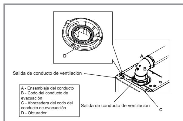
figura 14 - Obturador de pared
