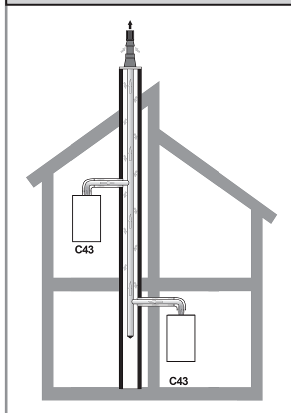
figura 21 - Posibilidades de conexión (tipo C43)
