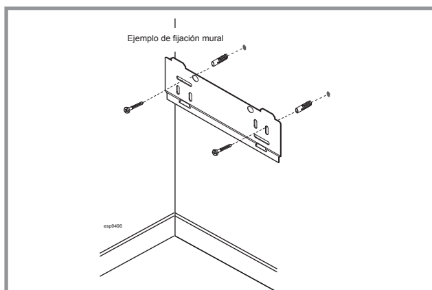
figura 8 - Preparación de la instalación en el muro
