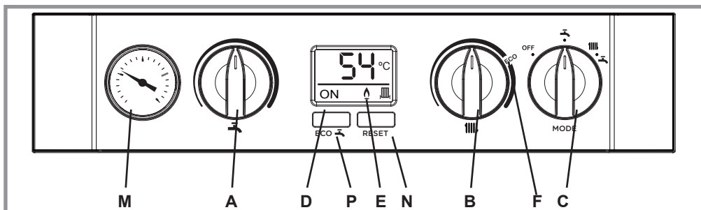
figura 37 - Controles de funcionamiento
