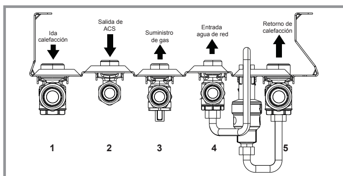
figura 31 - Conexiones
