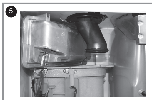
figura 45 - Incline el quemador
