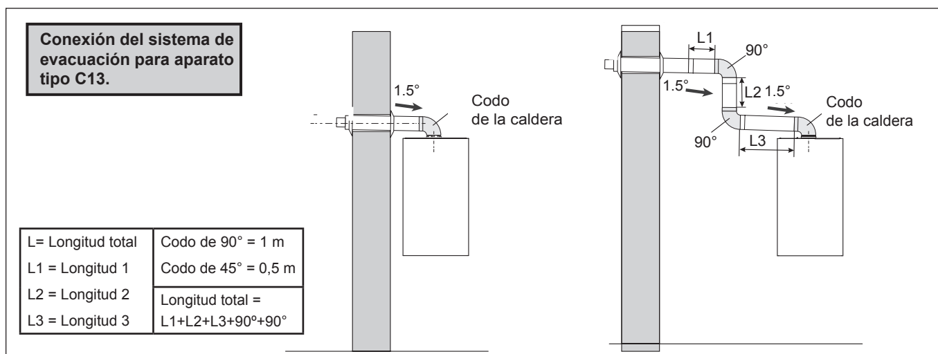
figura 18 - Instalación posterior del conducto tipo C13
