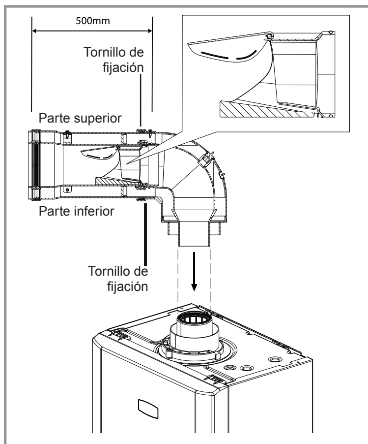
figura 20 - Conjunto de la válvula de retención (aparatos tipo C43)
