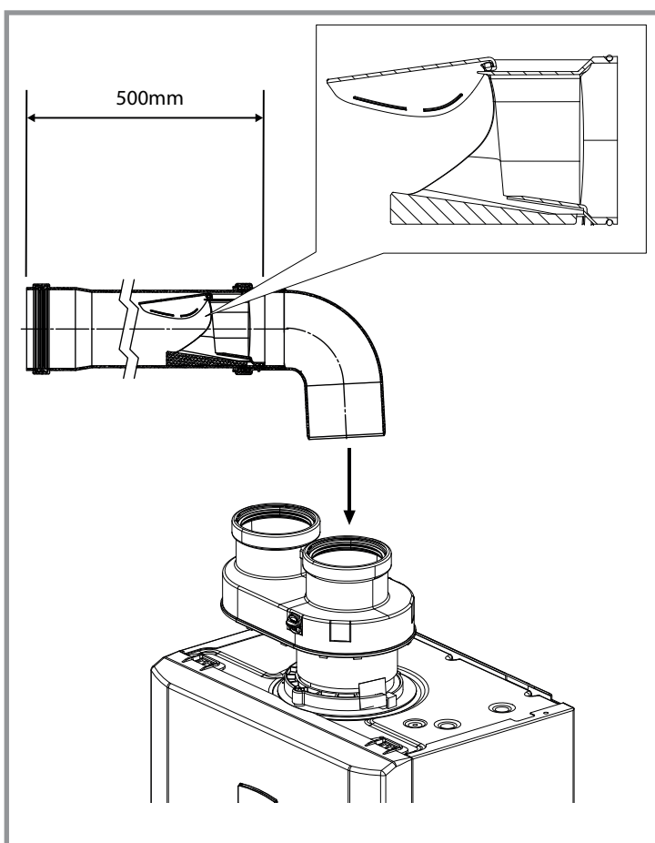
figura 24 - Conjunto de la válvula antirretorno (instalaciones tipo C83)
