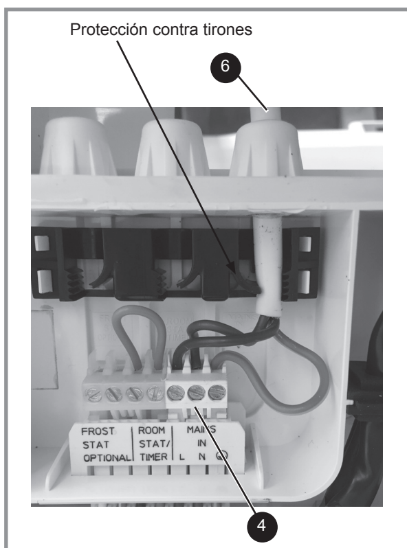
figura 35 - Cable de red preinstalado
