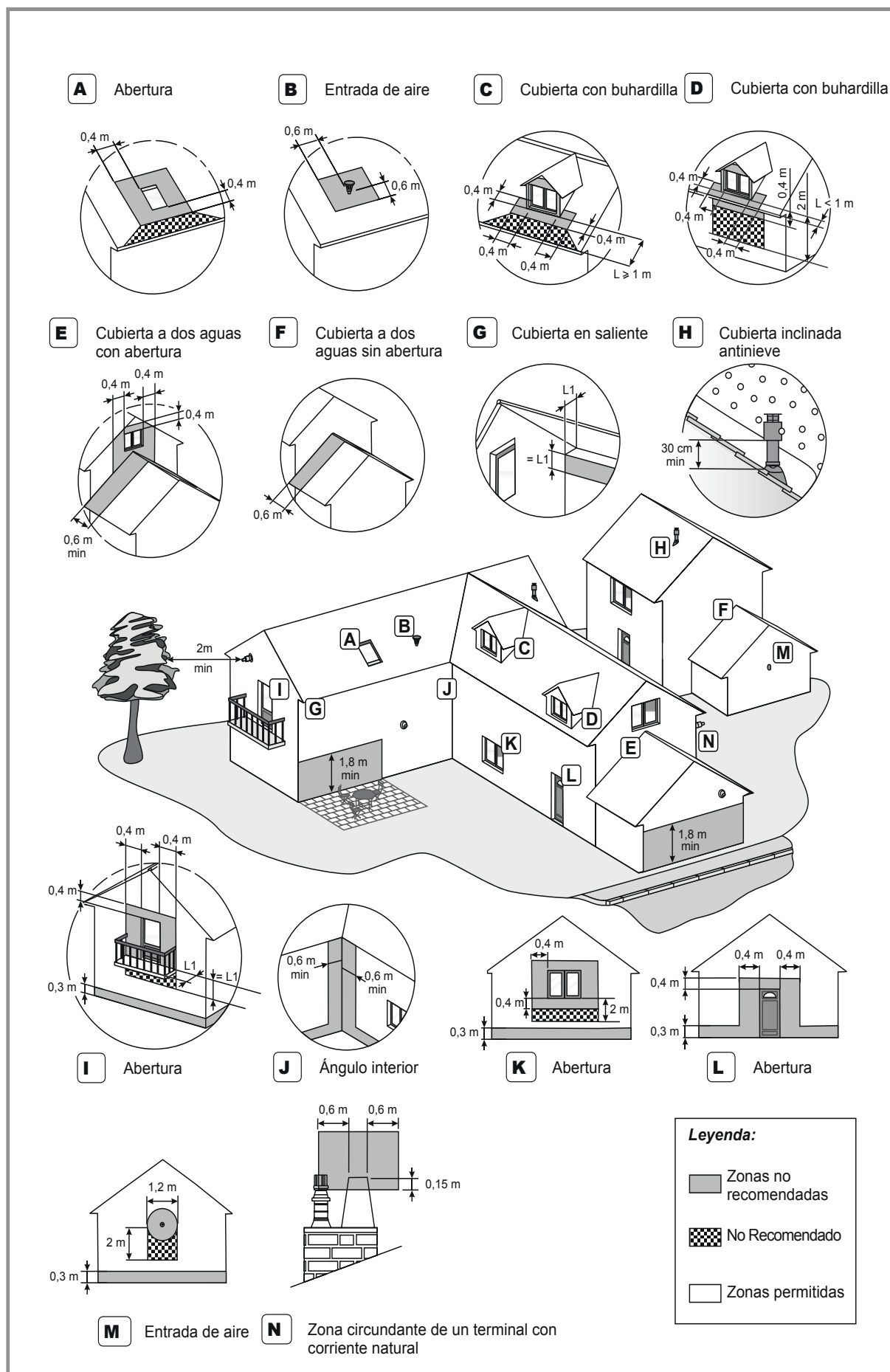
figura 29 - Normas para instalar los terminales sellados de una caldera de gas (tipos C13, C33, C43)
