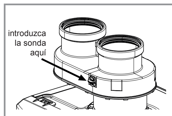
figura 26 - Medición de la presión del conducto (instalación tipo C83)
