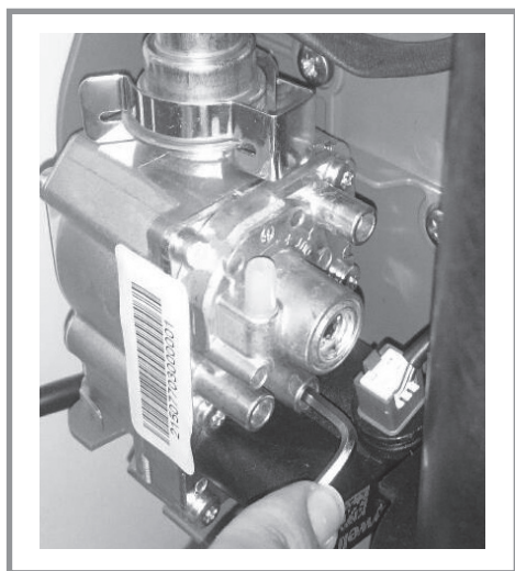
figura 36 - Entrada de presión del gas
