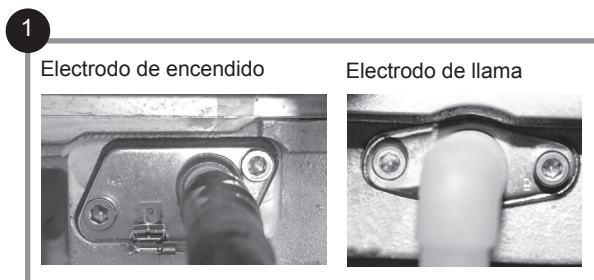
figura 47 - Electrodos de detección de llama
