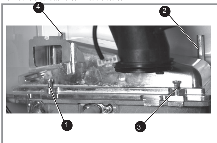
figura 49 - Reensamblaje del colector del conducto de evacuación
