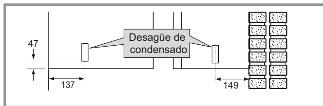
figura 30 - Ubicación del tubo de desagüe del agua de condensación
