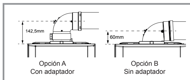
figura 15 - Opciones de instalación tipo C13
