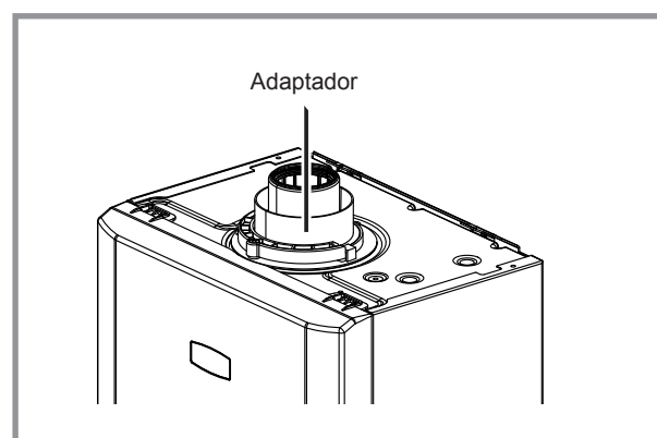
figura 12 - Instalación del adaptador
