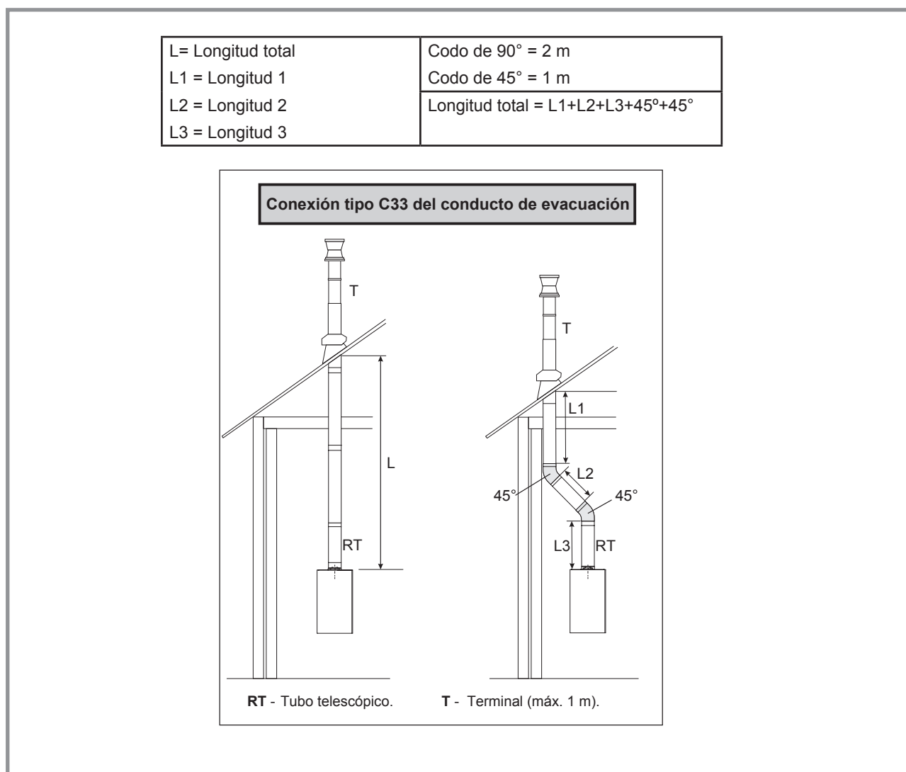
figura 19 - Posibilidades de conexión (tipo C33)
