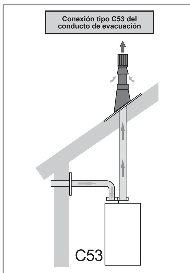
figura 23 - Posibilidades de conexión (tipo C53)
