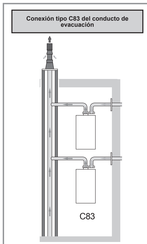
figura 25 - Posibilidades de conexión (instalación tipo C83)
