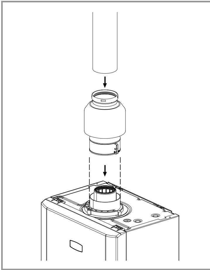
figura 27 - Montaje del conducto ( configuración B23P)
