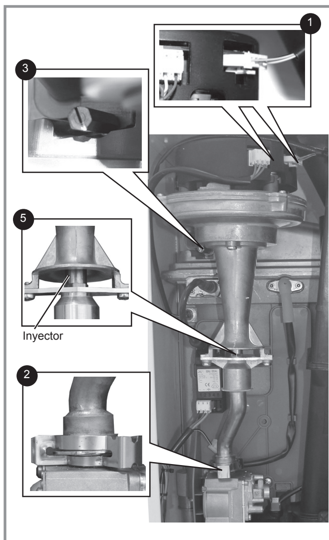
figura 42 - Retirada del ventilador y del tubo Venturi
