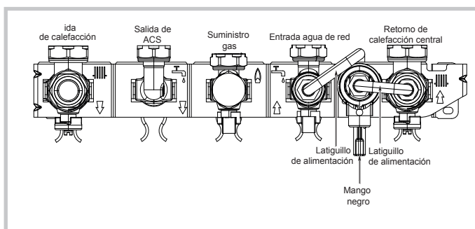
figura 32 - Conexiones del latiguillo de alimentación
