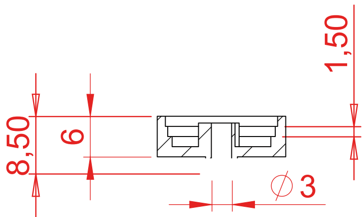
SECCIÓN A-A
