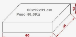
Lastre para Solarbloc de 28° a 34°
