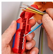
Retirar el aislamiento de conductores individuales
