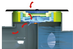
Válvula de aireación abierta Válvula de respiro abierta
