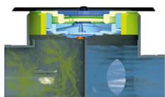
Válvula de aireación abierta Válvula de respiro abierta
