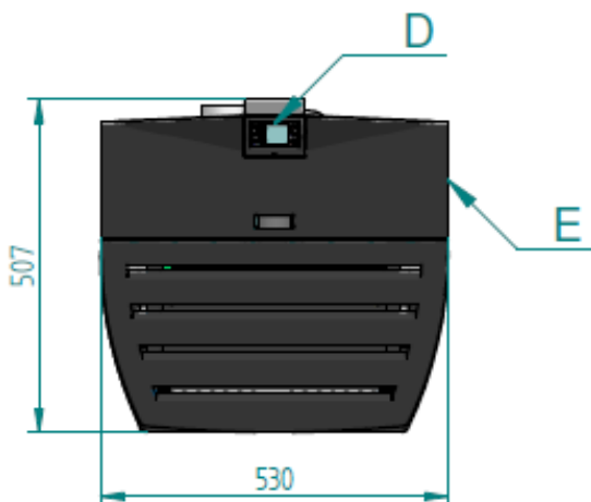
Ingombri stufa pellet VENUS
