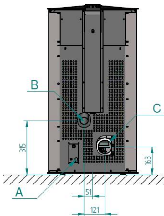
Medidas de la estufa de pellets VENUS
