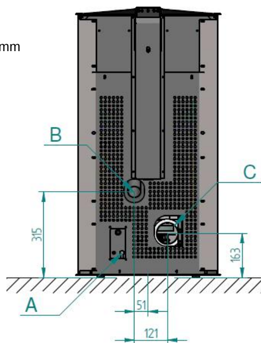
Dimensions du poêle à granulés VENUS
