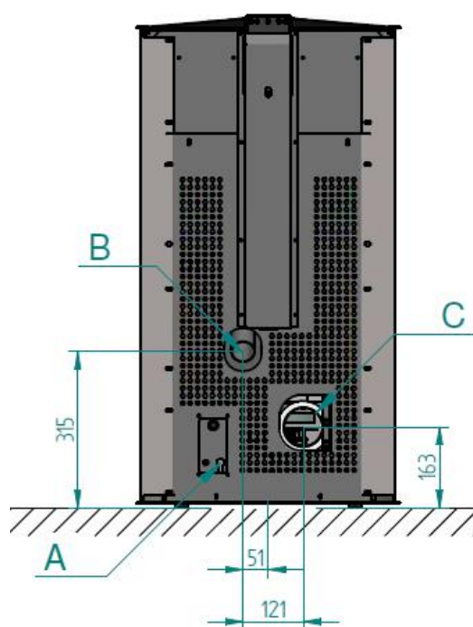
Abmessungen Pelletofen VENUS
