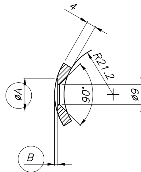
Sezione B-B
