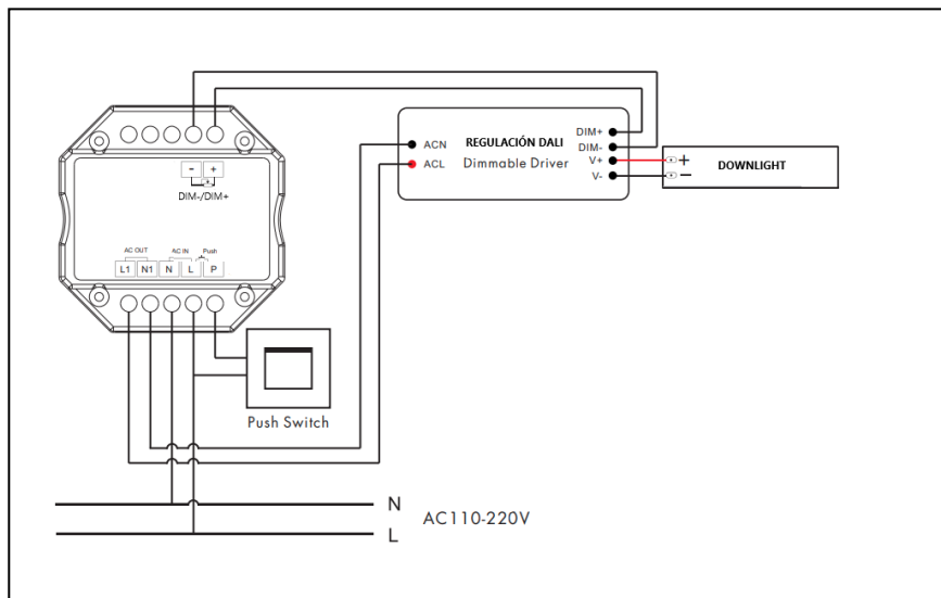
REGULACIÓN DALI
