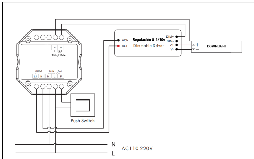
REGULACIÓN 0-10V
