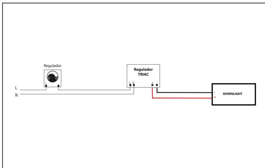
REGULACIÓN TRIAC
