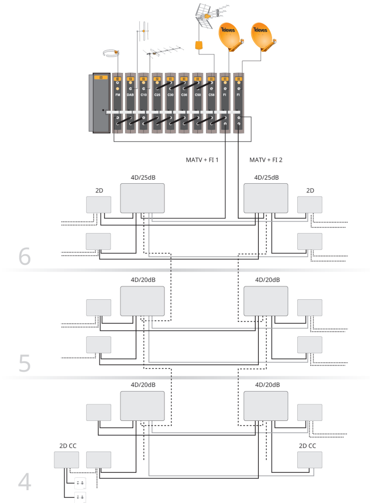
Red de distribución y Red interior de usuarios.
