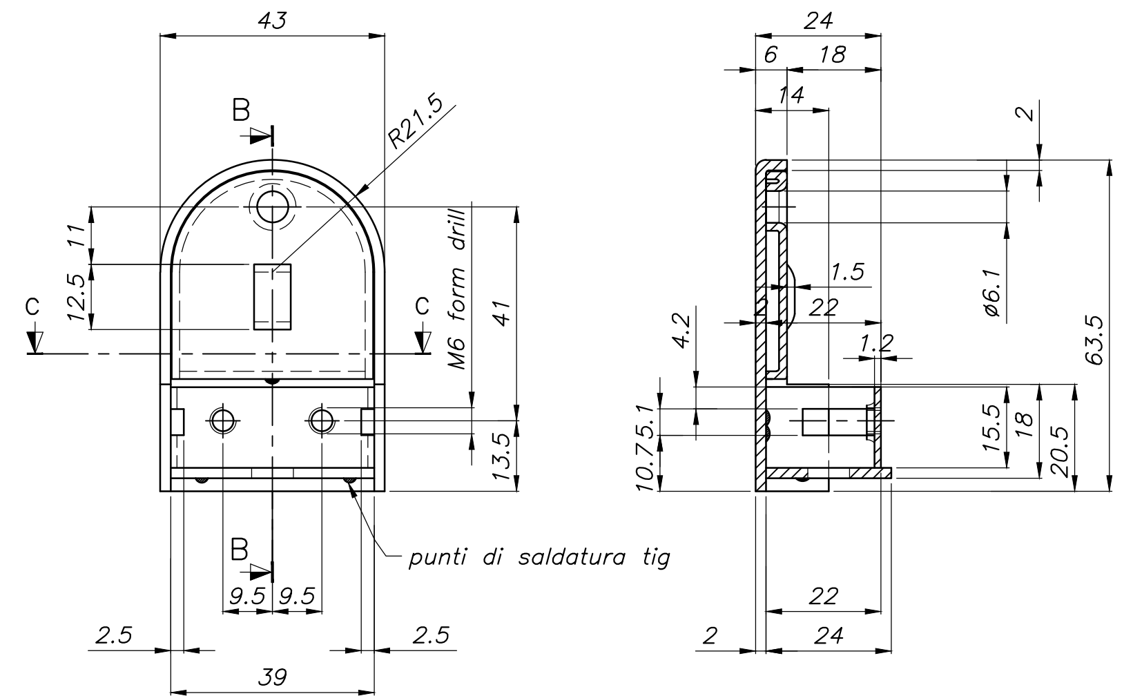
SEZIONE B-B
