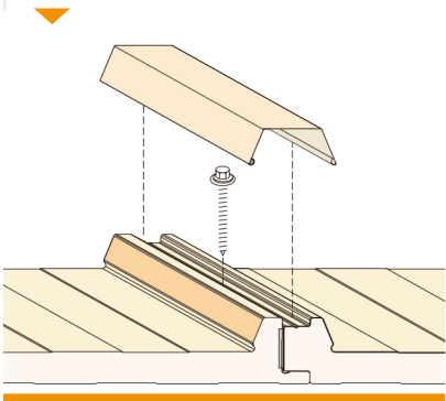
Detalle de junta.
