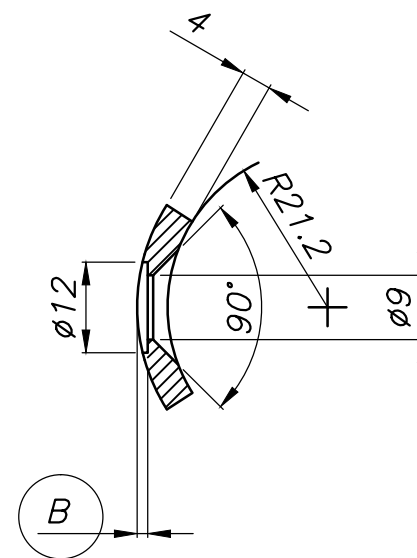
Sezione B-B
