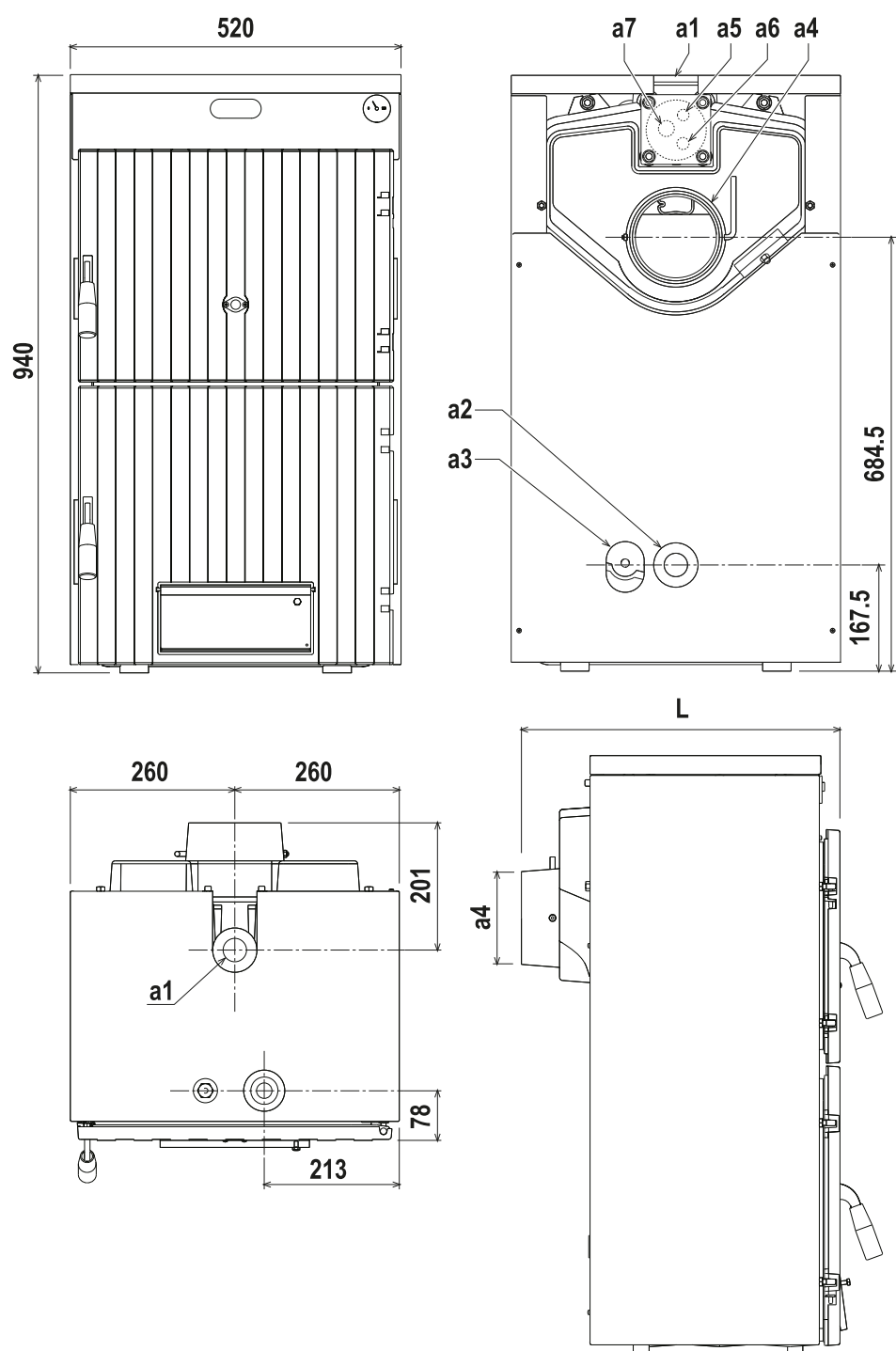
fig. 17 - Dimensiones y conexiones
