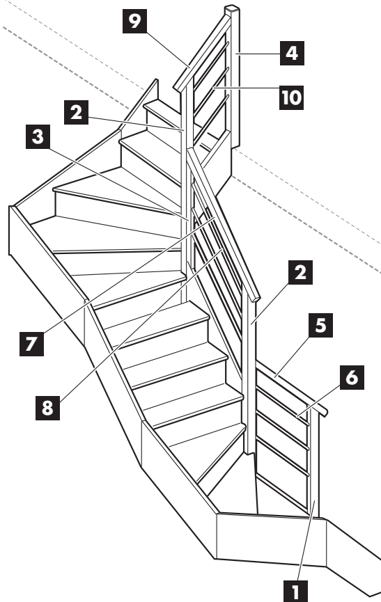
Exemple : Vue générale - 2 quartiers intermédiaires tournant à droite avec contremarche - rampe à Tubes
