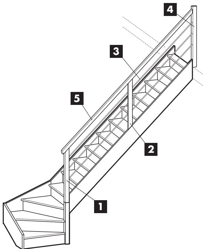
Exemple : Vue générale - 1 quartier bas tournant à droite avec contremarche - rampe à Tubes
