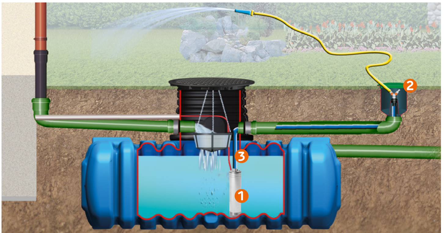
Exemple d'installation avec une cuve FLAT (Cuve + filtration vendues séparément)
