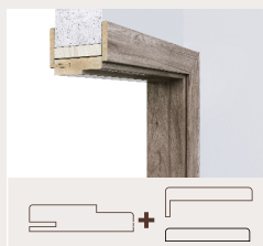
Cerco SRE Moldura TEX+TR2 MDF Encolado con cola PUR
