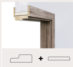
Cerco SR2 Moldura TR2 60/70/90 x 20 mm (medidas cerco) MDF Encolado con cola PUR
