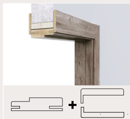
Cerco SRE Moldura TEX 1/2 70/90/110/130 x 30mm (medidas cerco) MDF Encolado con cola PUR
