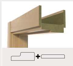
Cerco SR2 Moldura TR2 Cerco MDF Hidrófugo Moldura MDF Hidrófugo Encolado con cola PUR
